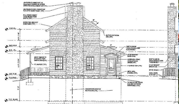
4 RIGHT ELEVATION
