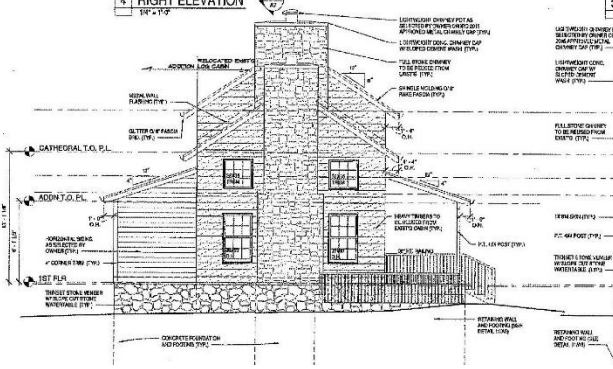
4 RIGHT ELEVATION
